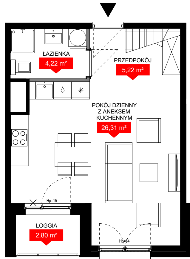
PIĘTRO 11
