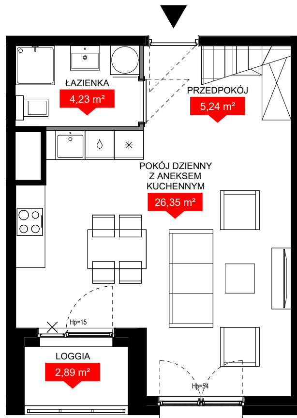
PIĘTRO 12
